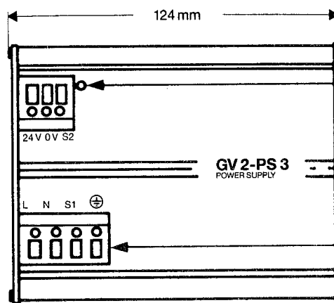
Frontansicht / Front view / Vue de face Vista frontale / Vista de frente
