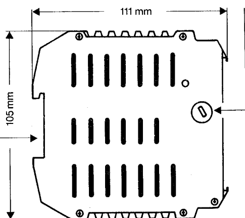
Seitenansicht / Side view / Vue de côté Vista lateral / Vista de lado
