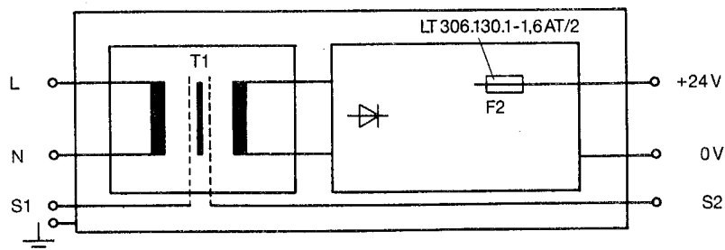
Blockschaltbild / Block diagram / Schéma fonctionnel / Schema / Esquema de conexión
