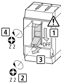
1b NZM.2...
